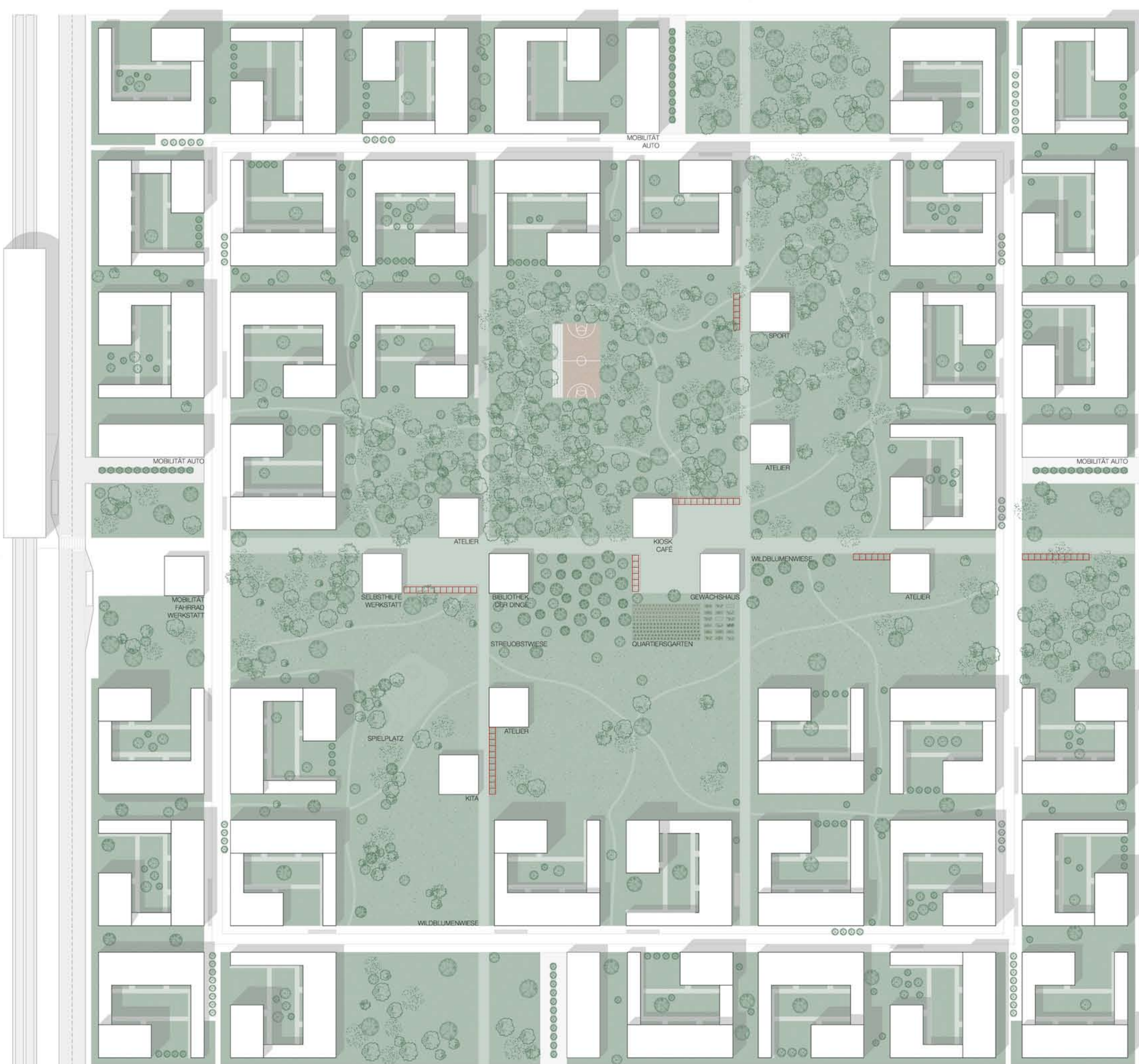
LAGEPLAN MS 1:1000
