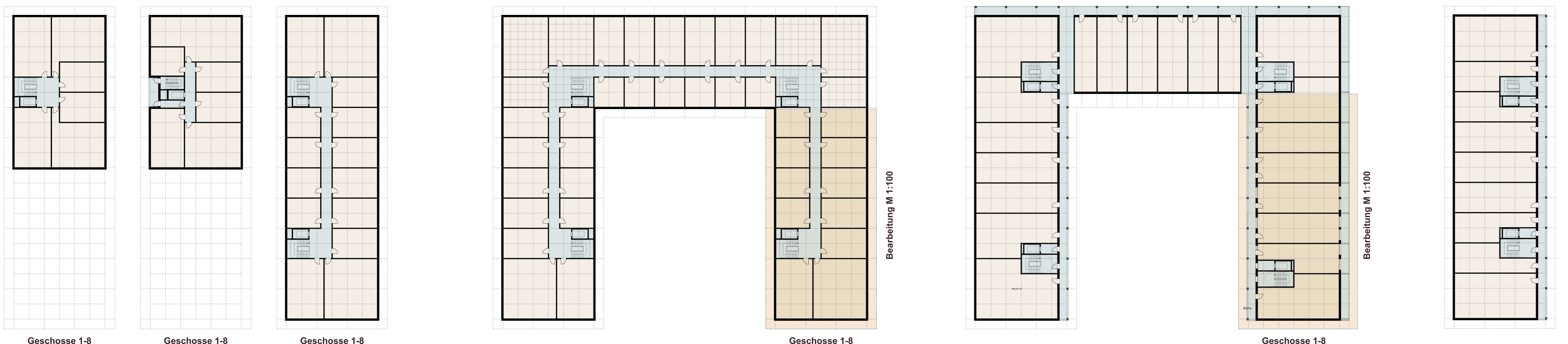
Grundrisse Mittelgang M 1:100
