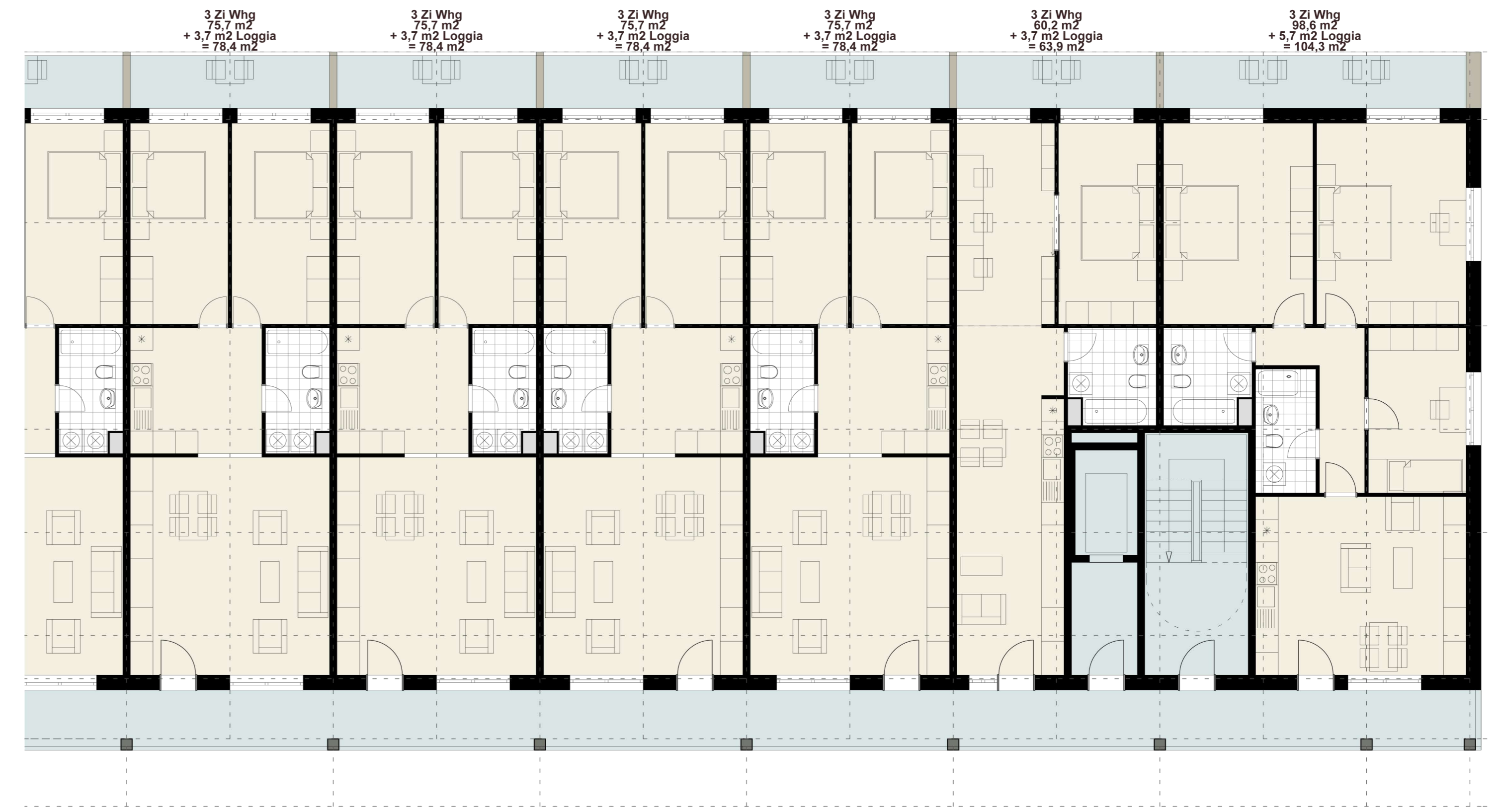
Grundrisse Laubengang M 1:100
