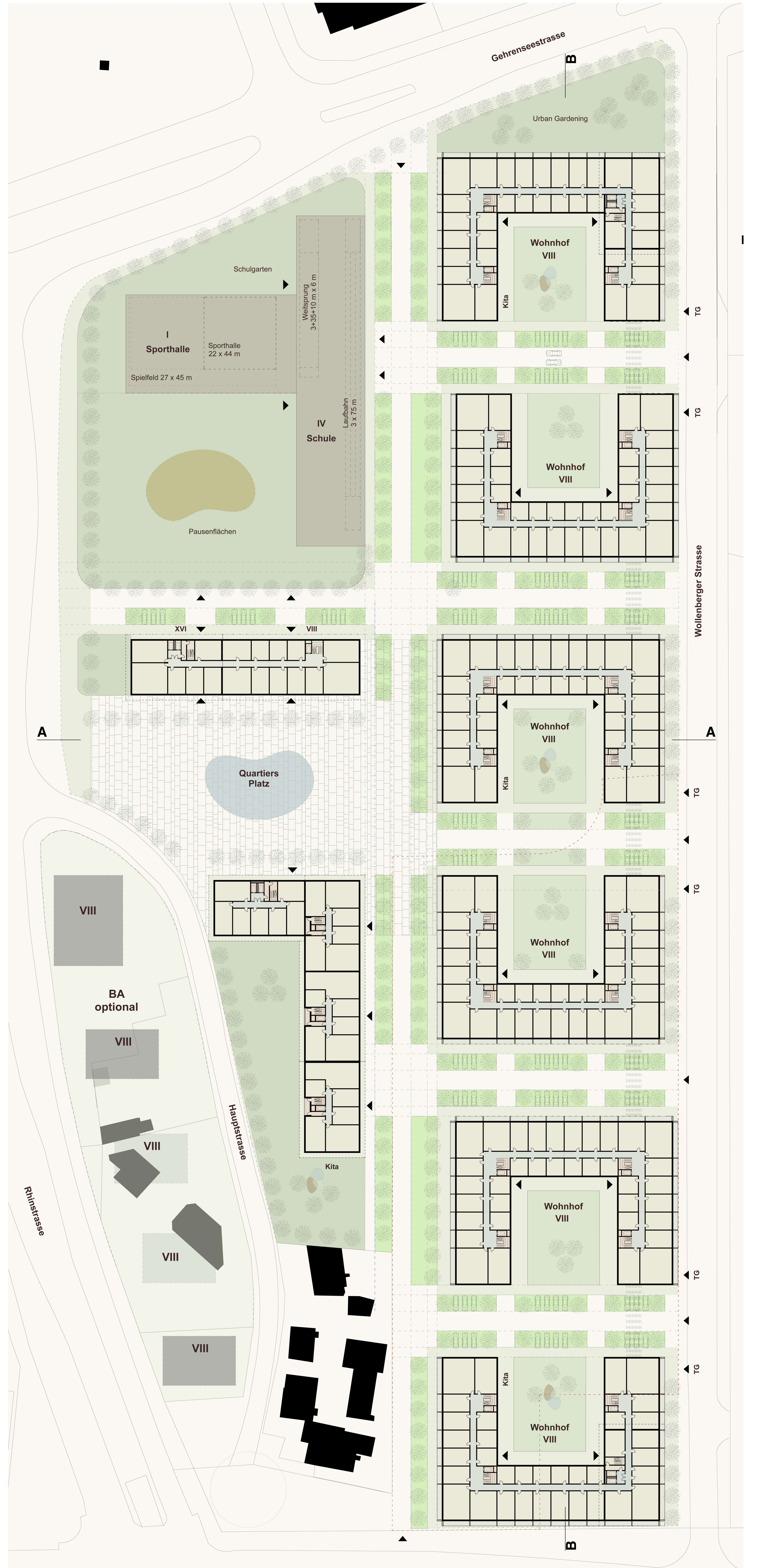
Regelgeschoss M 1:500
