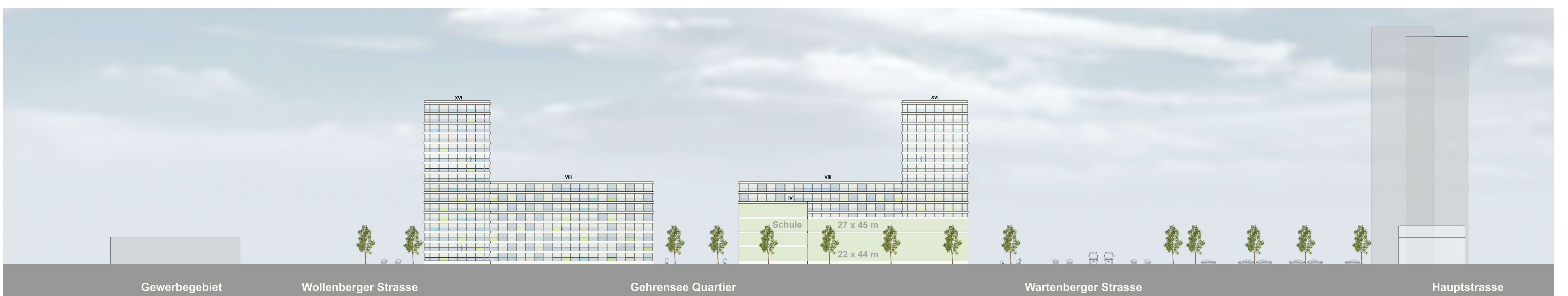
Ansicht Norden / Gehrenseestrasse M 1:500
