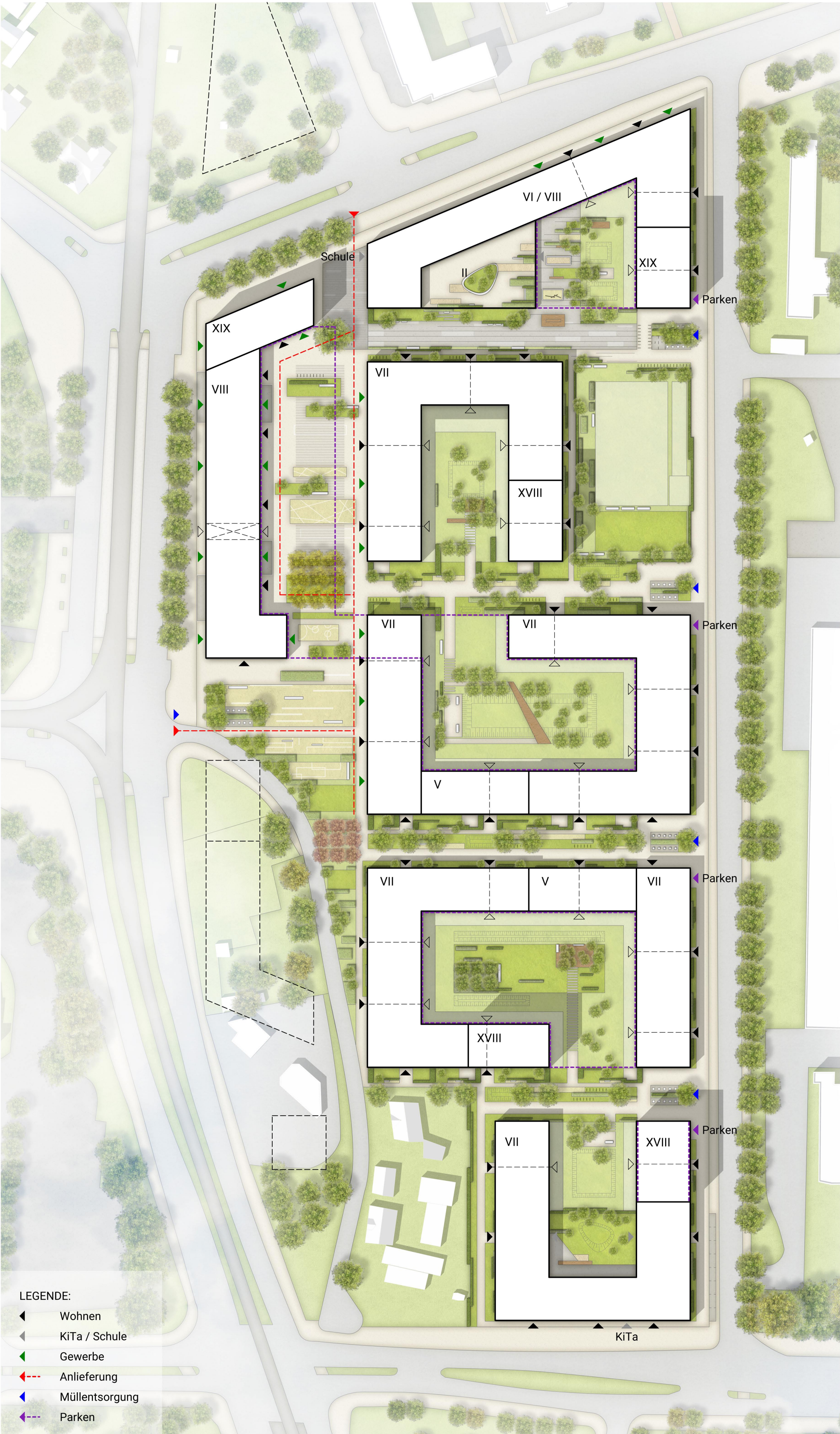
ERSCHLISSUNG 1:1000
