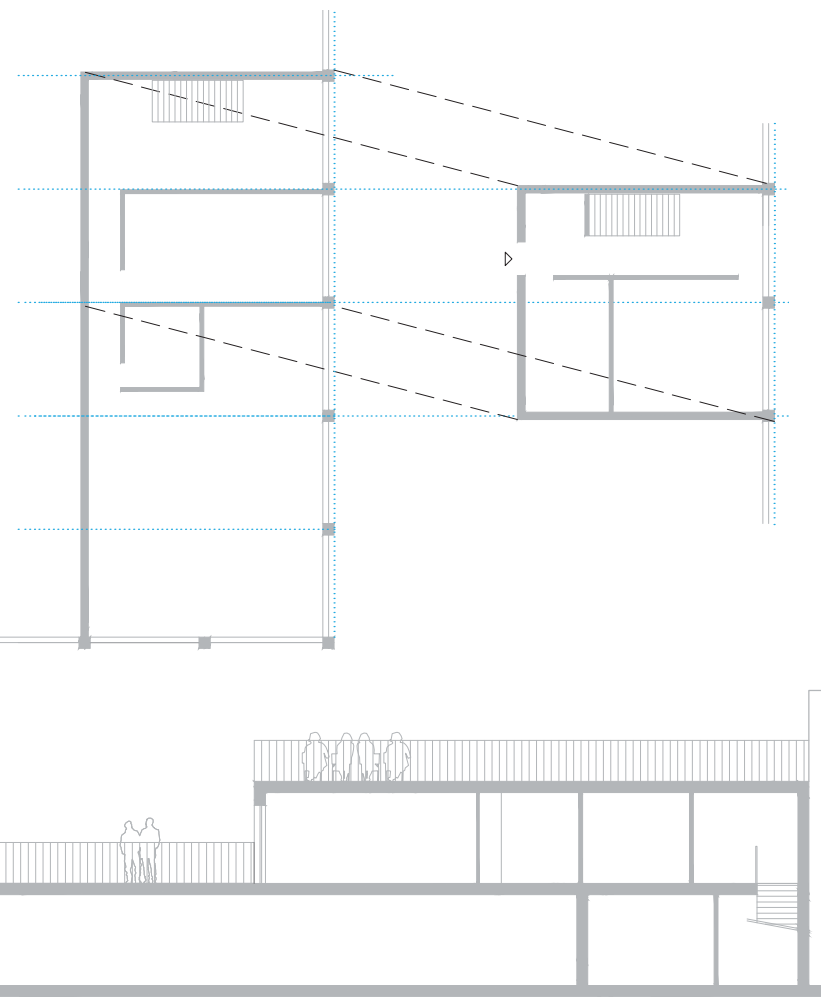
VARENTA - TERRASSE DUPLEX 1:200
