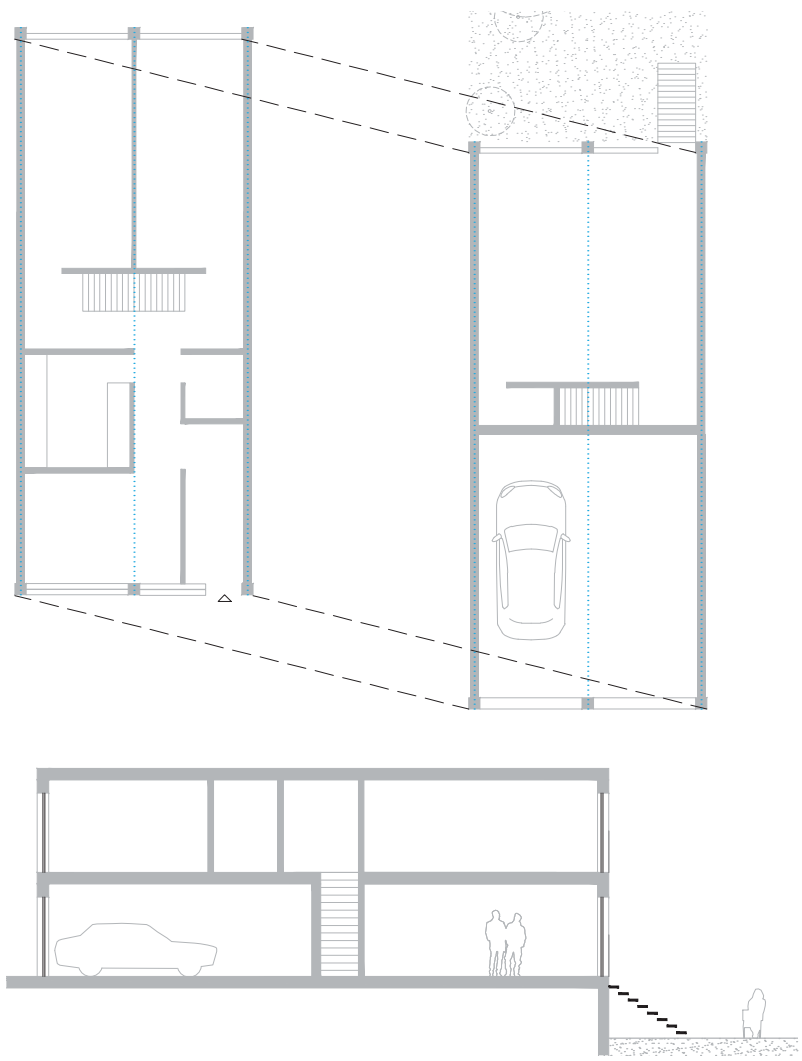
HOWOGE - T4 DUPLEX EG 1:200
