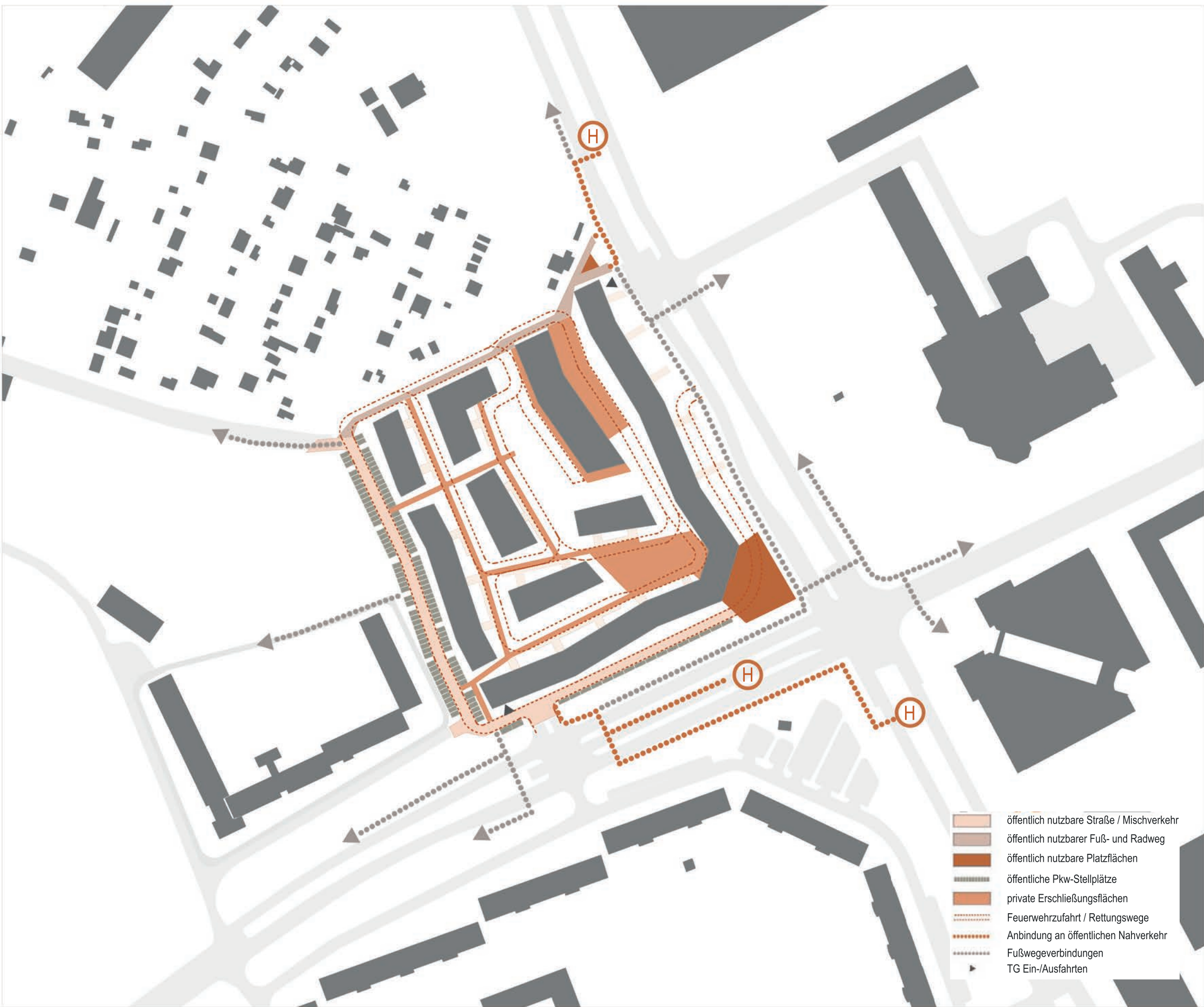
Erschließung Quartier 1:2000
