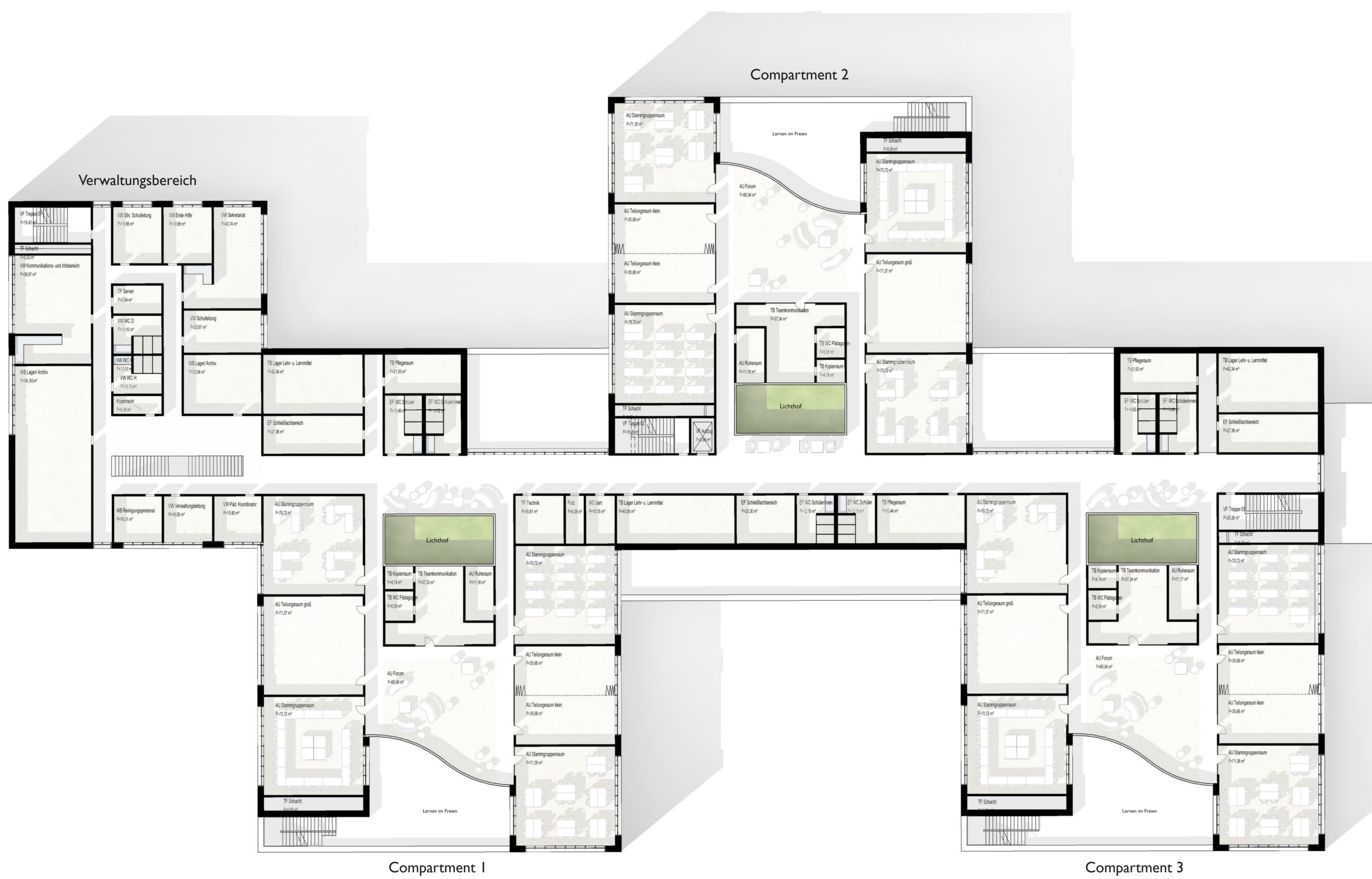
Grundriss OG1 1:200
