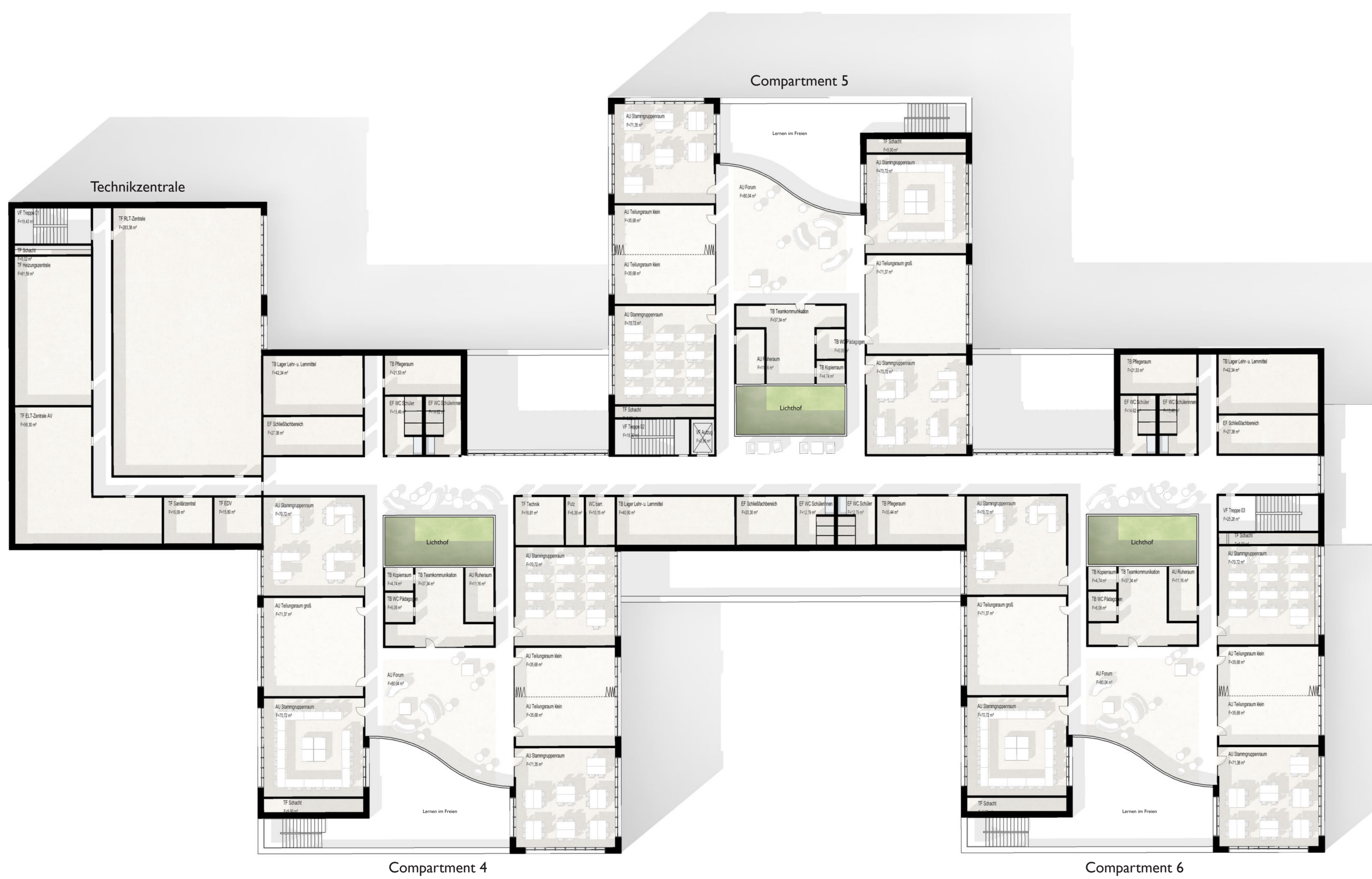
Grundriss OG2 1:200
