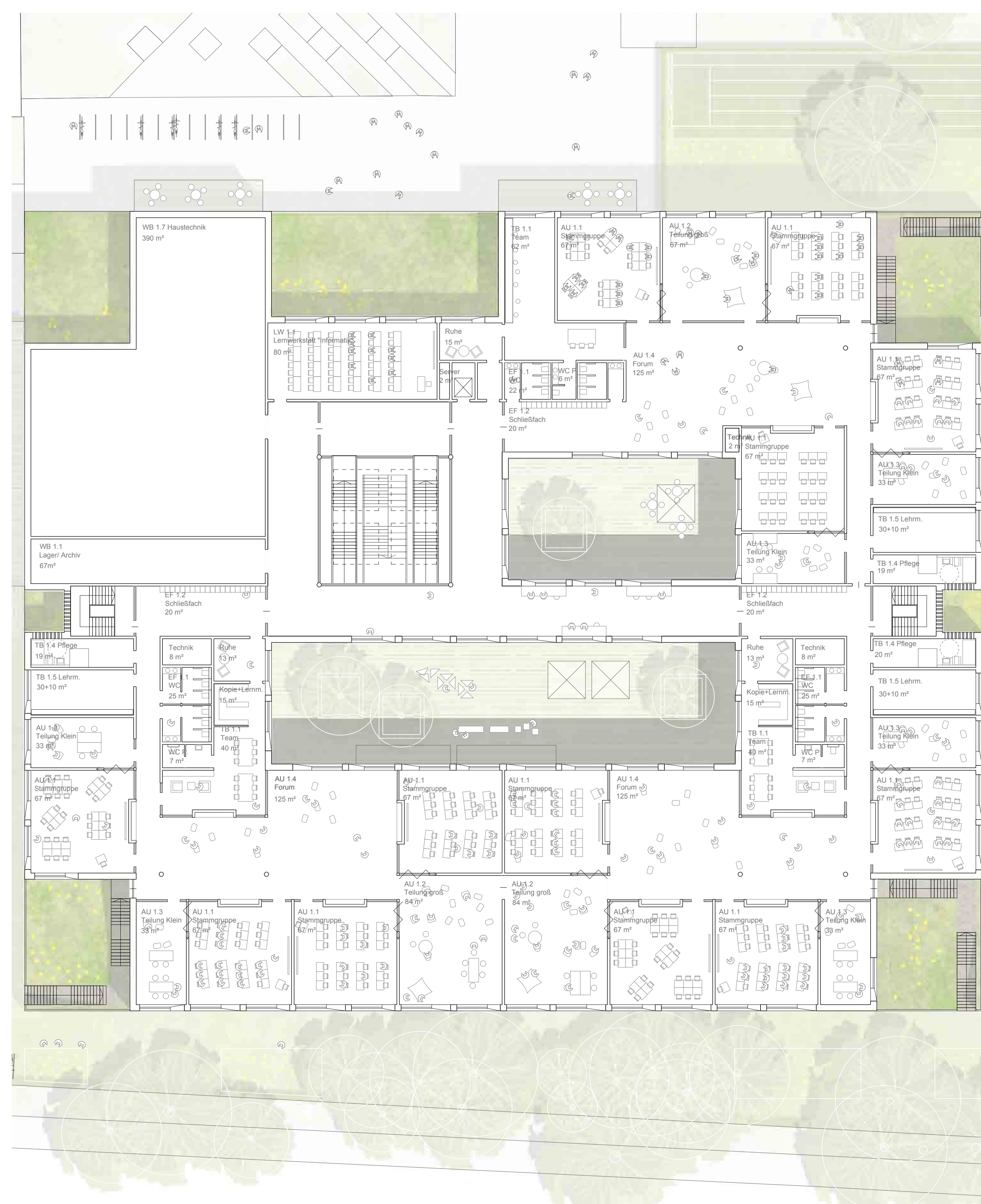
2. Obergeschoss Schule | M 1:200
