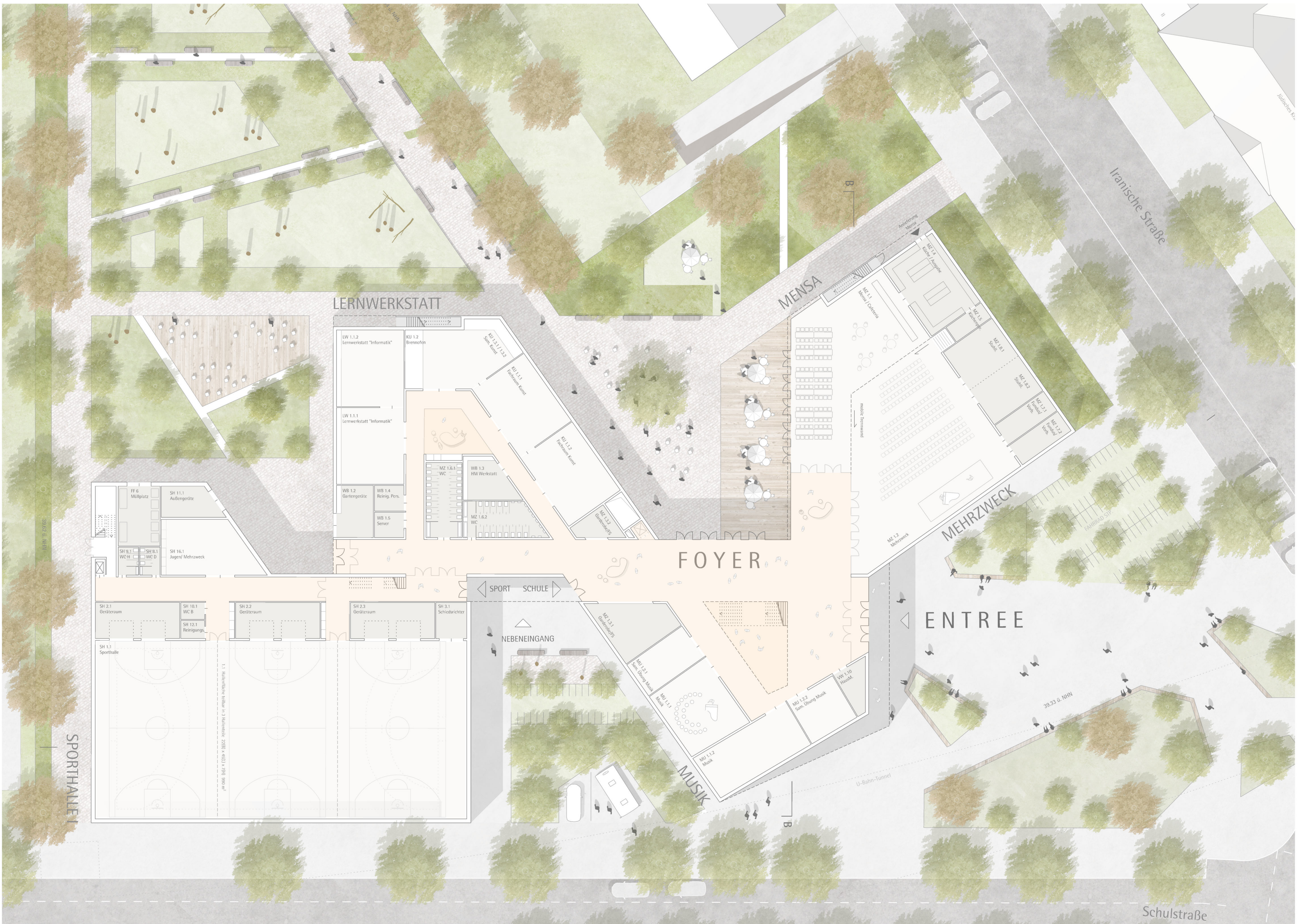
GRUNDRISS ERDGESCHOSS MIT AUSSENANLAGEN M 1:200
