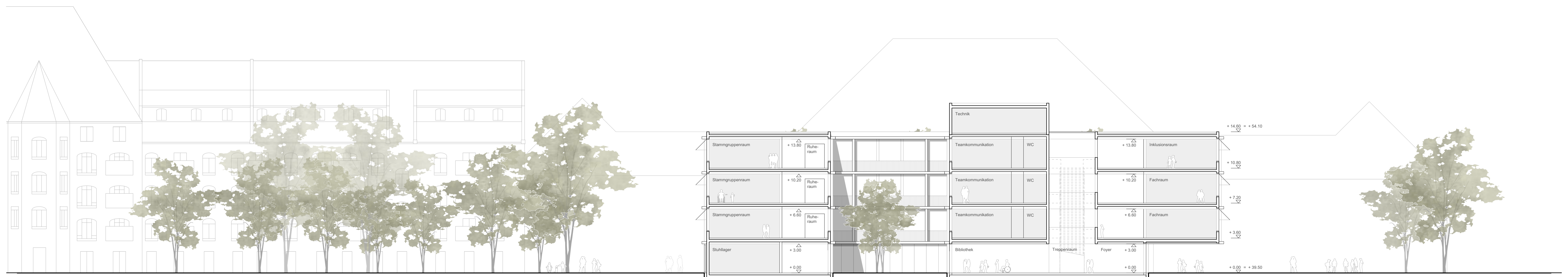
Schnitt A-A M 1:200
