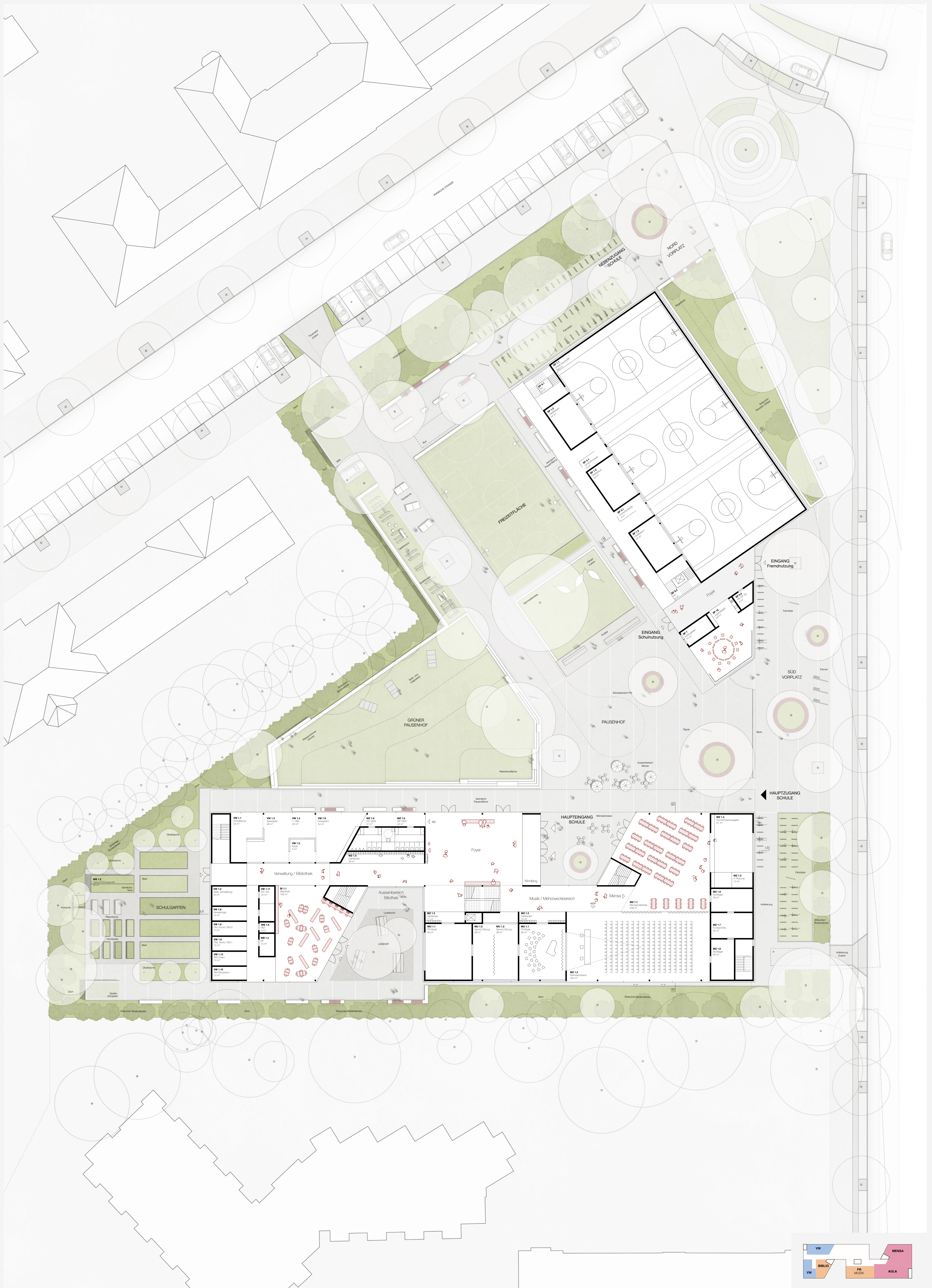
Grundriss Erdgeschoss M 1:200
