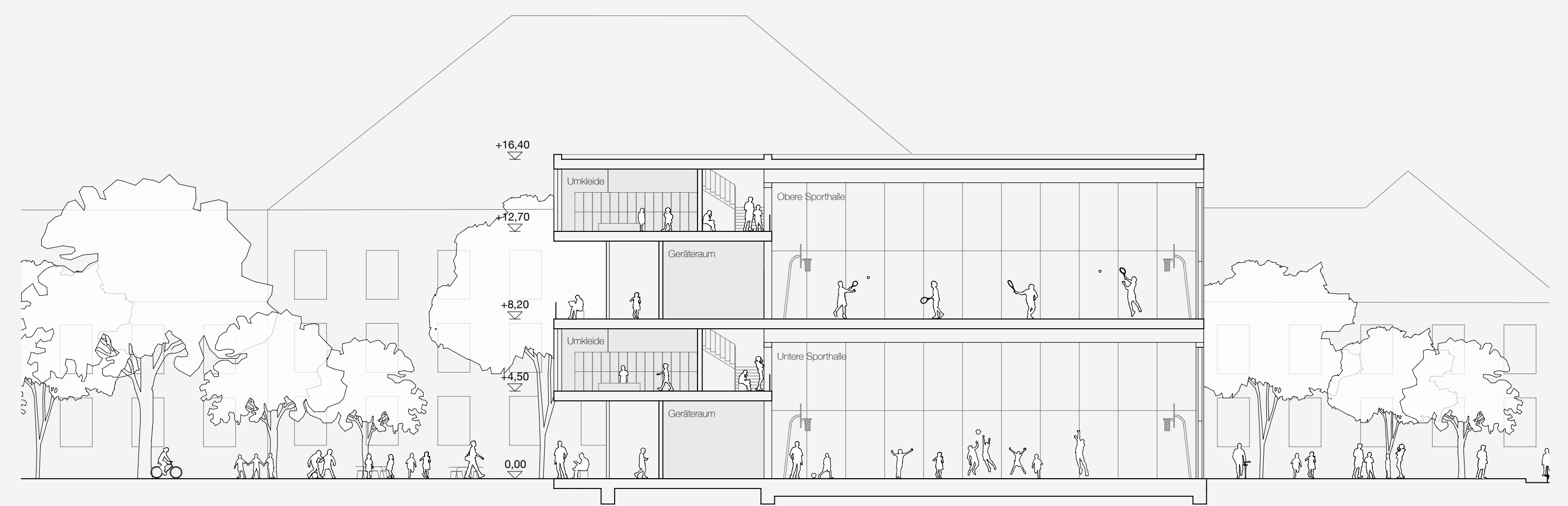
Querschnitt Turnhalle
