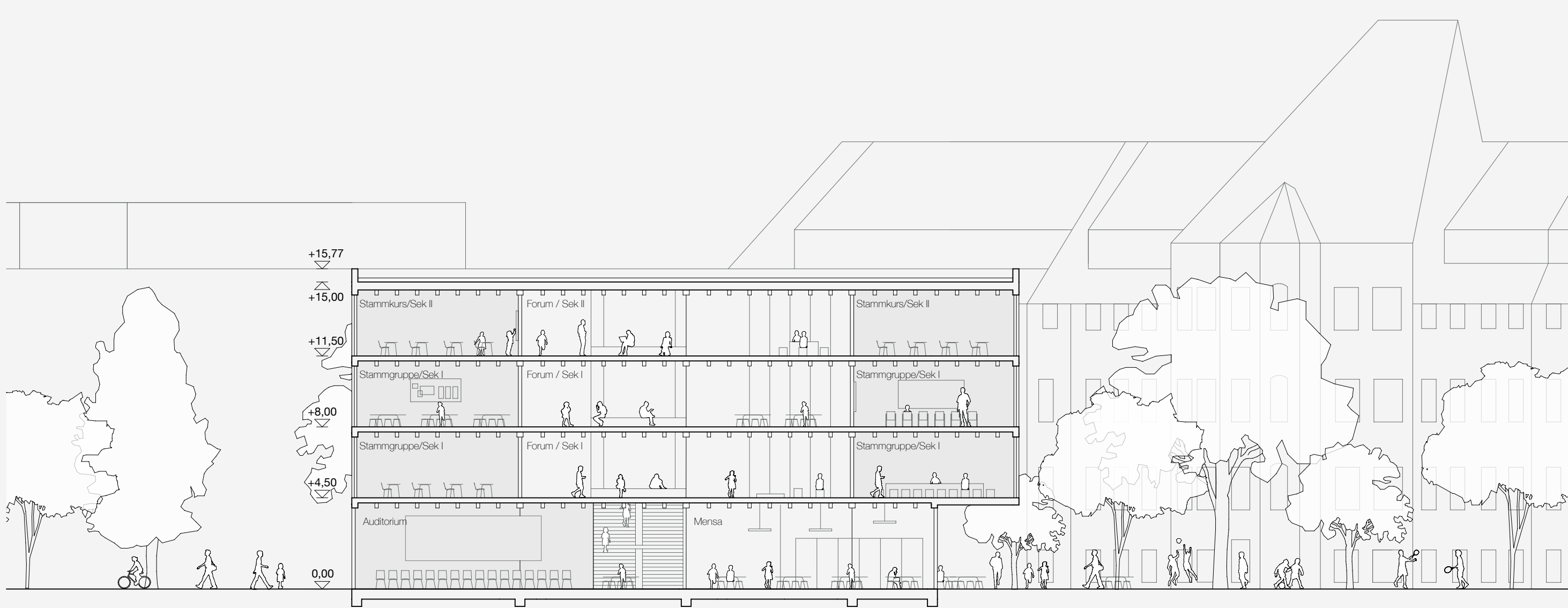
Querschnitt Gymnasium
