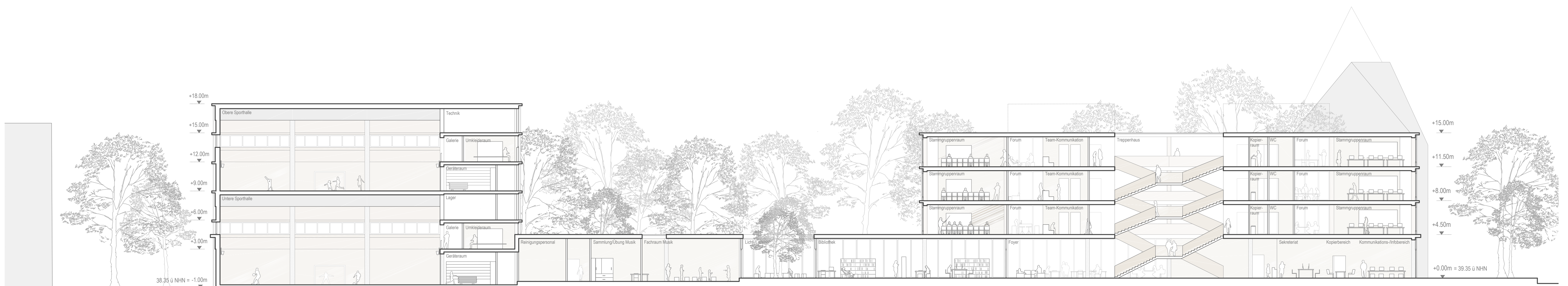
SCHNITT AA 1:200
