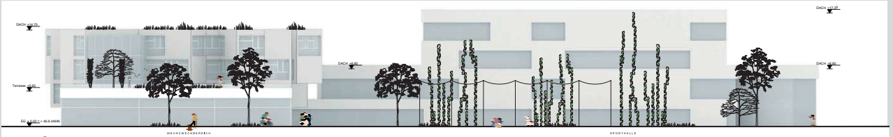
ANSICHT SÜD - 1:200
