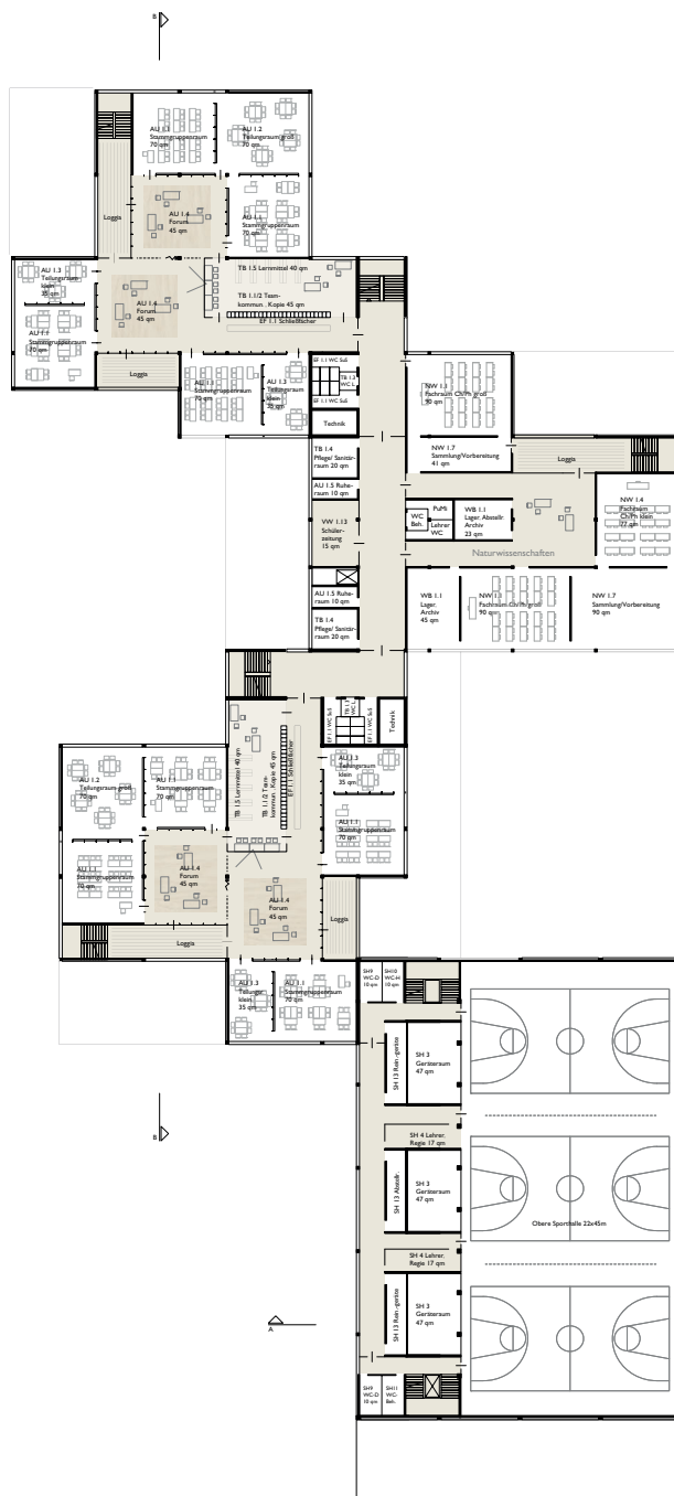
Grundriss 2.OG 1:200
