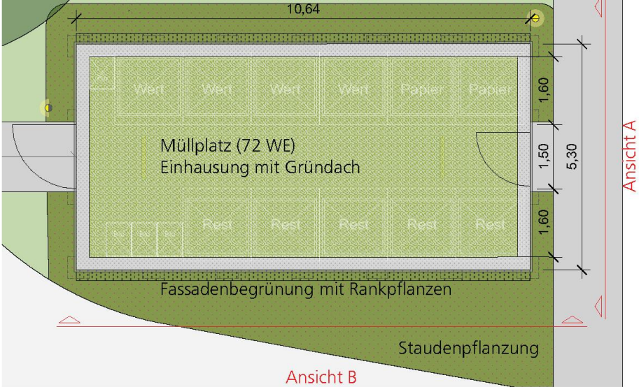
Ausschnitt Lageplan: Mülleinhausung überdacht, M 1:100
